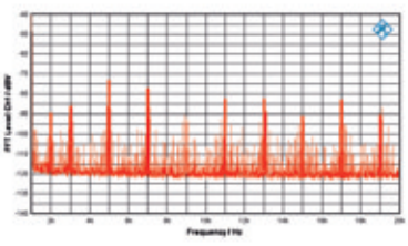
Klirrspektrum: Sugden Audio Fusion 21
