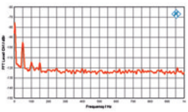
Störspektrum: Sugden Audio Fusion 21
